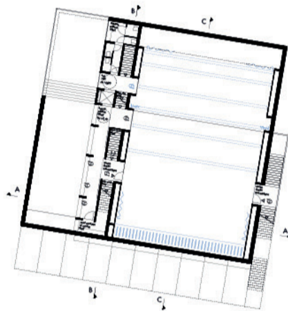
Plan 1er étage (grandin repâé) +2,70
