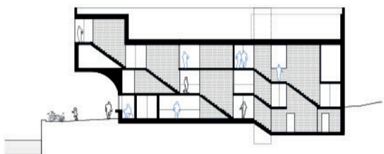
Coupe BB
