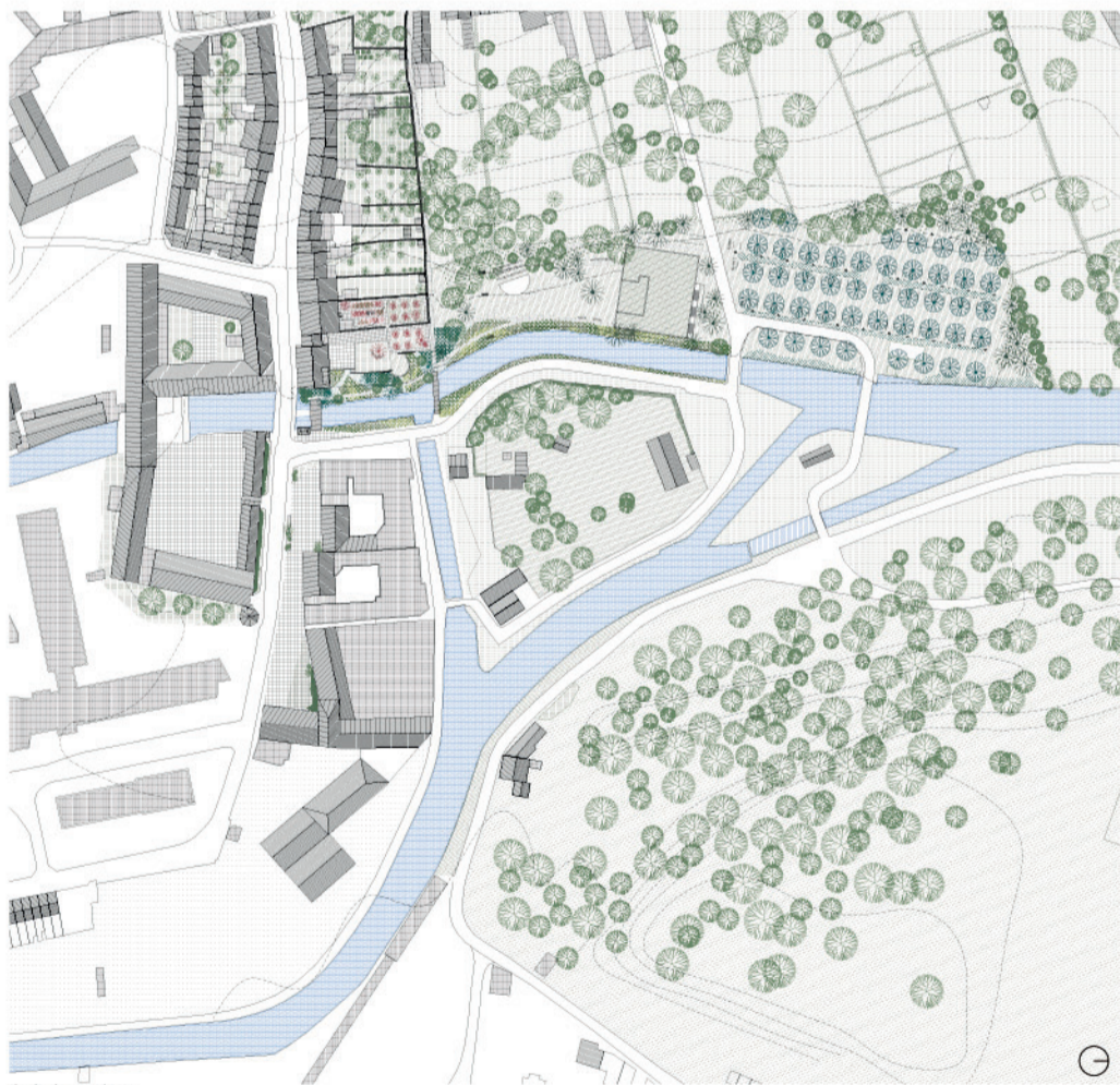
Plan d'implantation 1/1000e
