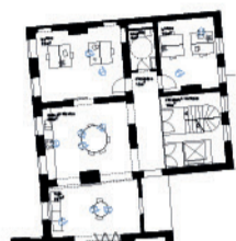
Plan 2e étage niv +5,80
