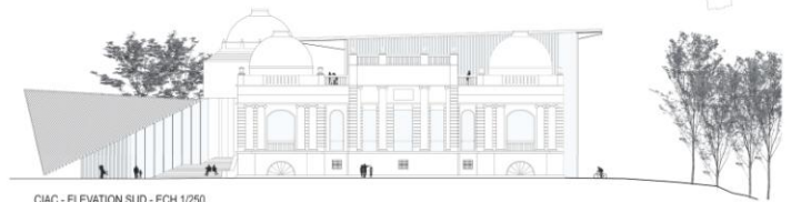
CIAC - ELEVATION SUD - ECH 1/250
