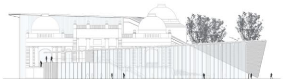
CIAC - ELEVATION NORD - ECH 1/250
