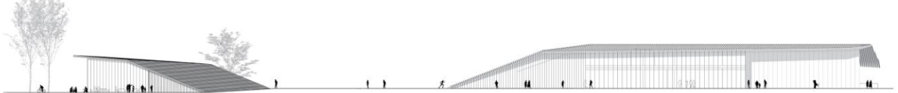
BRASSERIE, PAVILLON D'ACCUEIL, D'ESPACES PARTAGES - ELEVATION EST - ECH 1/250
