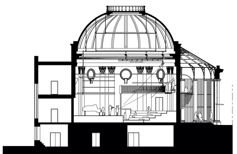
Coupe E
