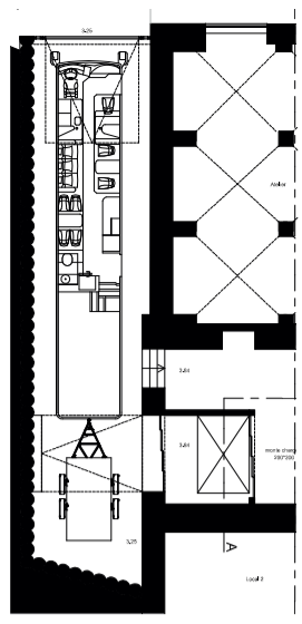
Plan R-1 (variante exigée)
