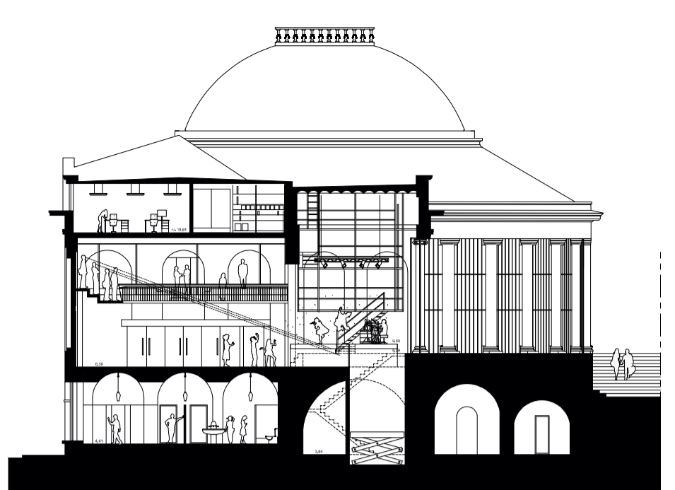
Coupe A
