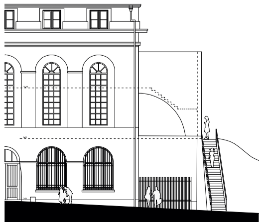
Elevation nord
