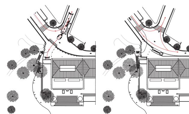
Implantation variante exigée 1/500
