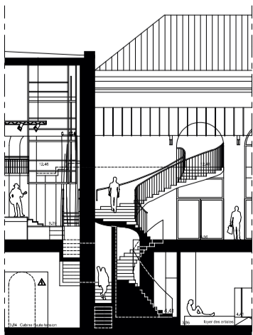
Coupe B
