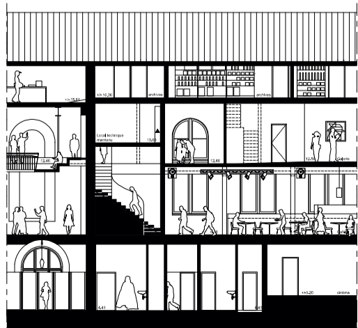
Coupe C
