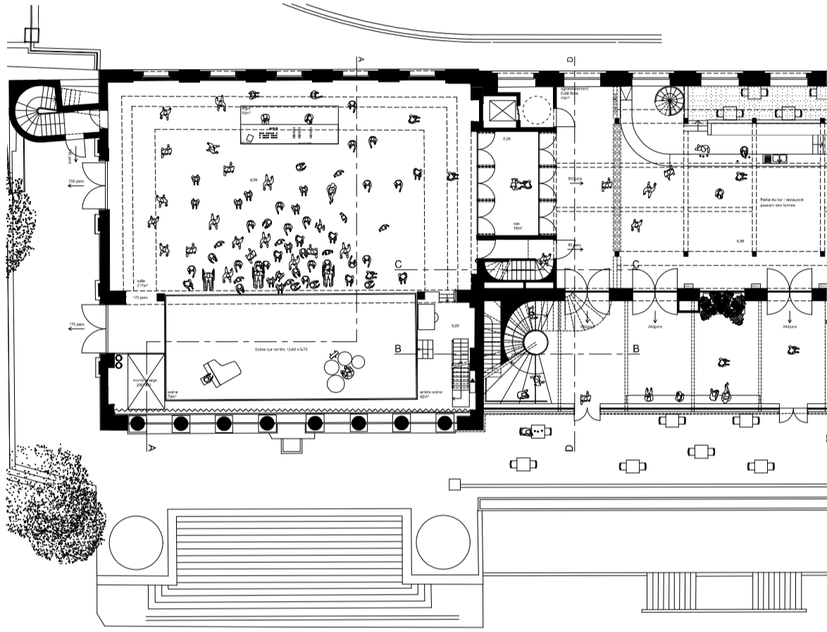
Plan Rez-de-chaussée
