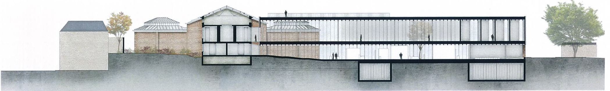
COUPE B
