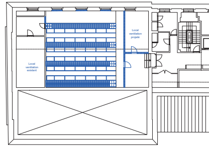
PLAN DU GRIL TECHNIQUE
