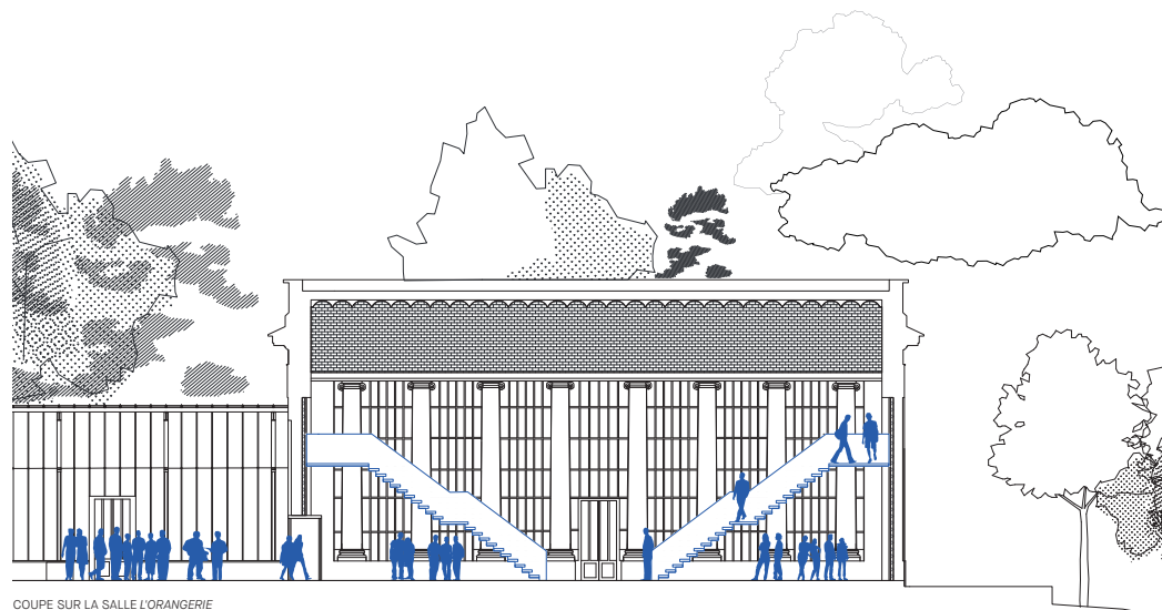
COUPE SUR LA SALLE L'ORANGERIE
