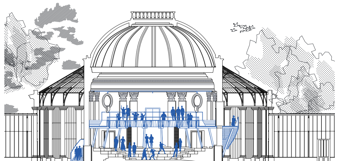
COUPE SUR LA SALLE LA ROTONDE
