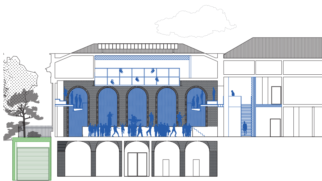
COUPE SUR LA SALLE L'ORANGERIE
