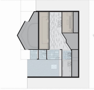
COUPE GRAND ESCALIER
