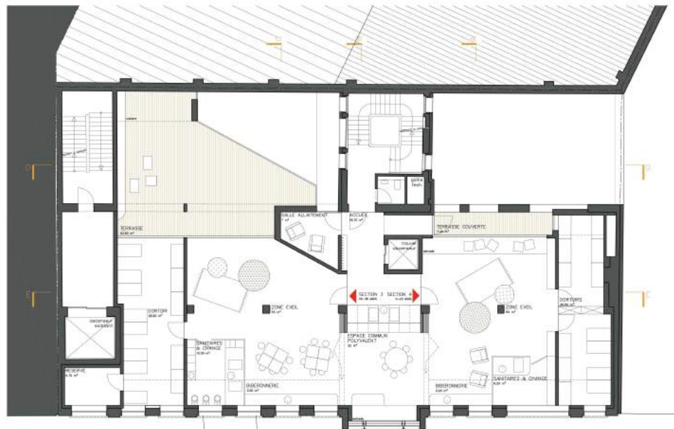
PLAN DU REZ +2 - échelle > 1/100
