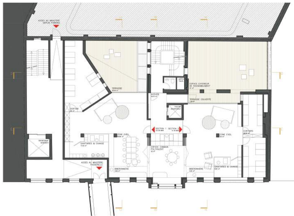
PLAN DU REZ +1 - échelle > 1/100
