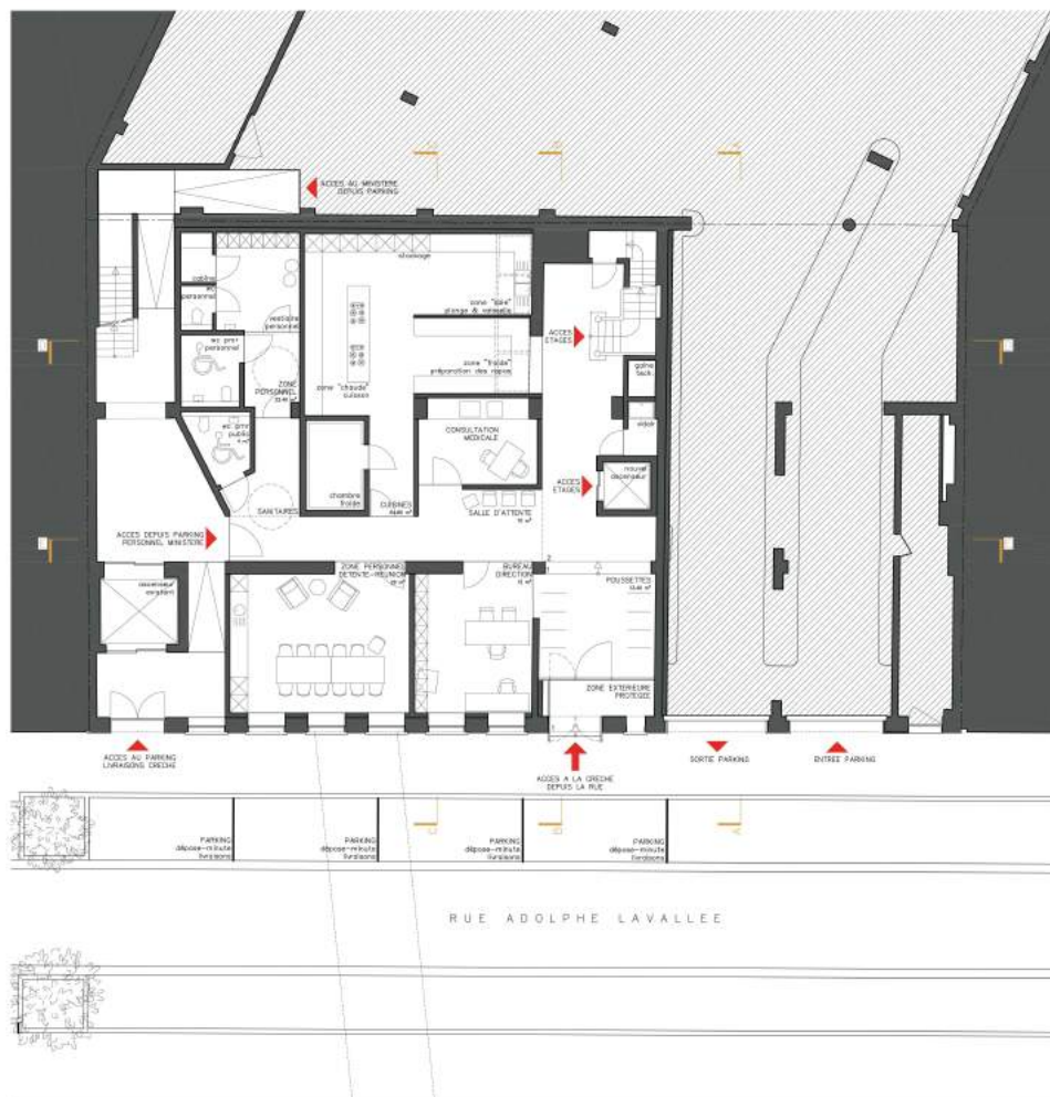
PLAN DU REZ-DE-CHAUSSEE - échelle > 1/100
